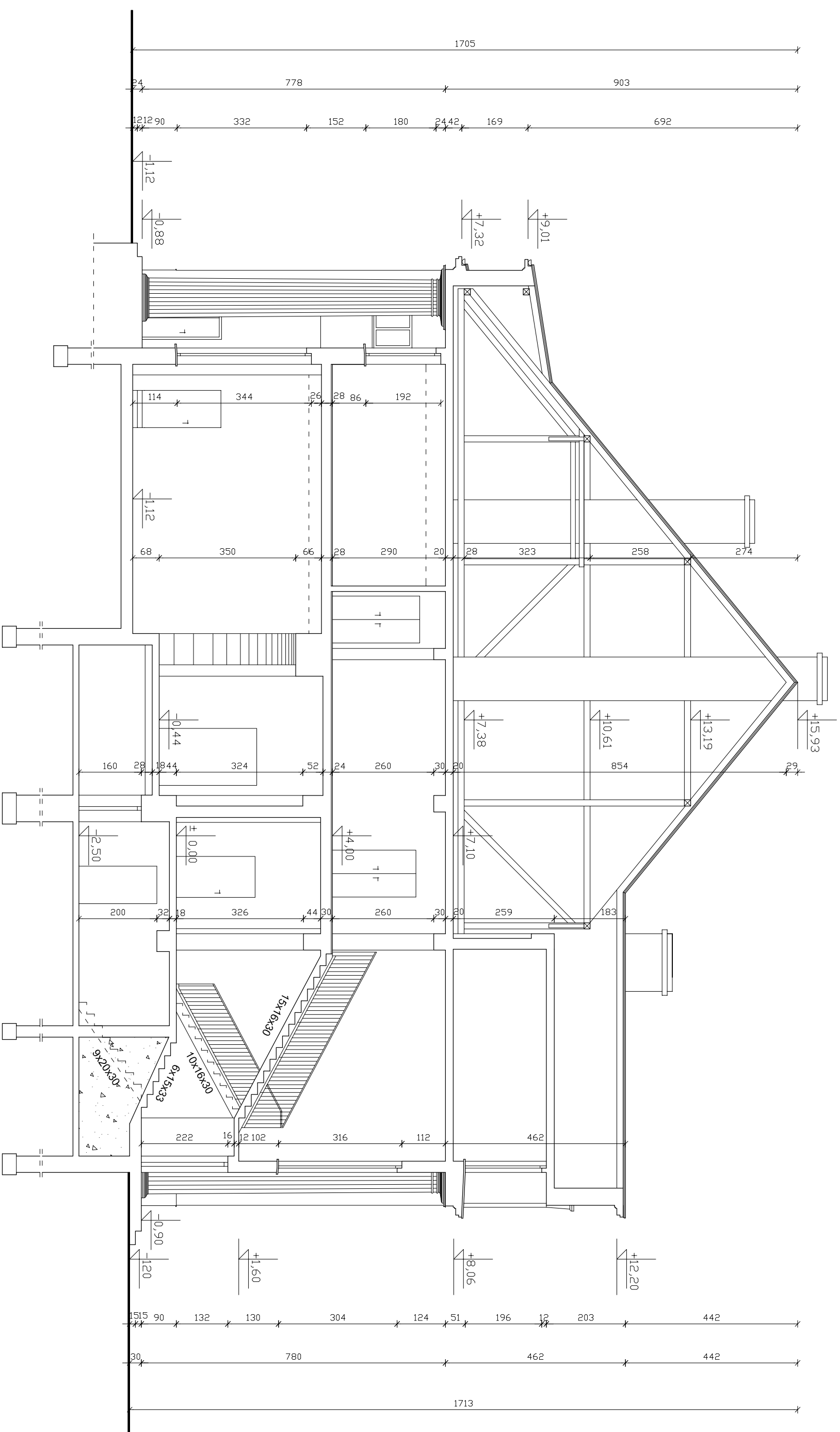
PRZEKROJ B-B Skala 1:100
