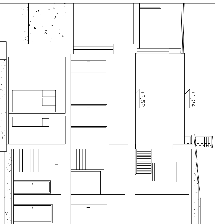
Przekroj A-A
