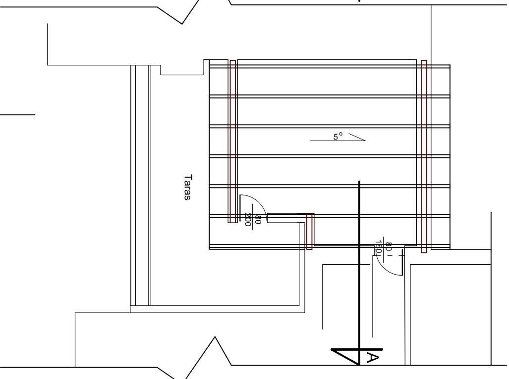
Rzut dachu
