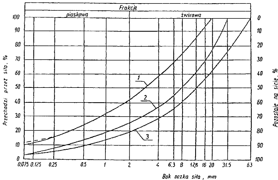
Rysunek 1. Pole dobrego uziarnienia kruszyw przeznaczonych na podbudowy wykonywane metodą stabilizacji mechanicznej 1-2 kruszywo na podbudow
