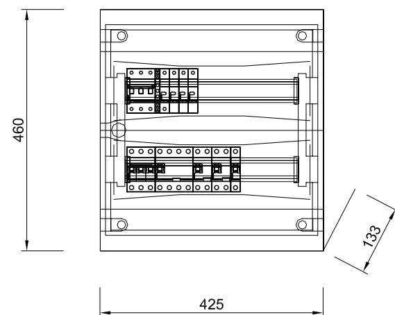
Rozdzielnica podtynkowa typu Ekinox TX, 2x18
