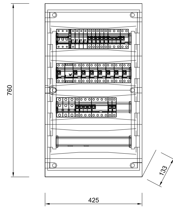
Widok 1:10
