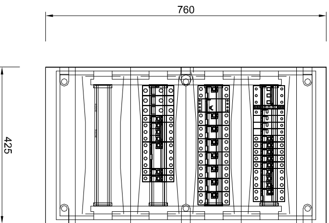
Widok 1:10
