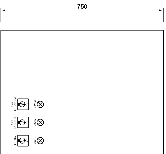
Widok 1:10
