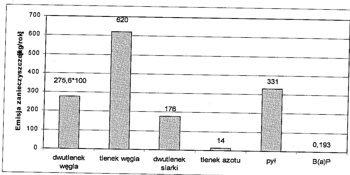
Rysunek 1. Emisję dla jednego obiektu mieszkalnego (obiektu standardowego)
